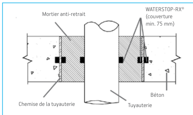
Finition de la tuyauterie chemisée
