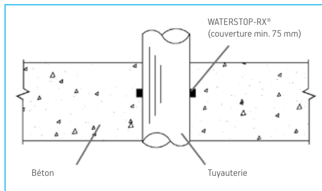
Corps passant crée lors de la coulée
